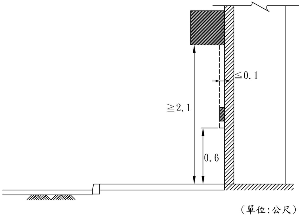
圖 6.2.1 人行道淨高限制參考圖
